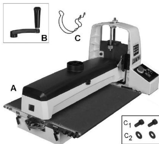
Figure 6-1: Ponceuse (JWDS-2550-M affiché)
