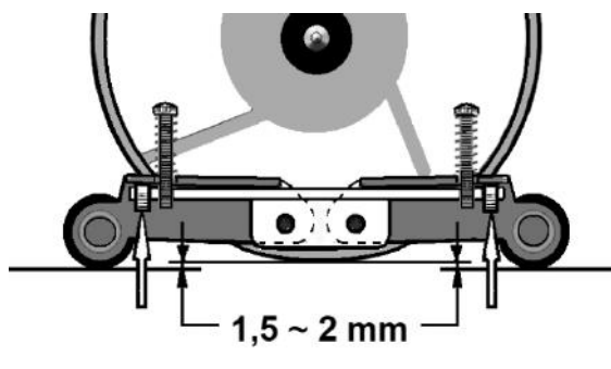
Abb. 8-6: Andruckrollenhöhe Stellschrauben
