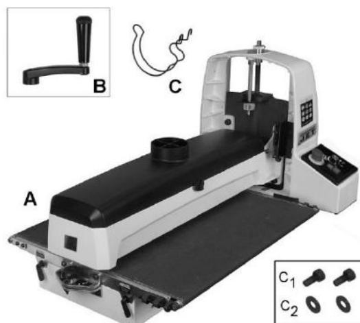
Abb. 6-1: Schleifmaschine (JWDS-2550-M abgebildet)
