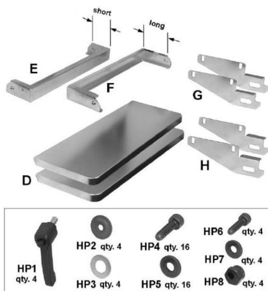
Abb. 6-2: Verlängerungstische (optional)
