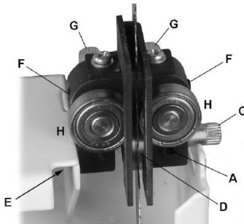
Abb. 26: Untere Sägeblattführungen
