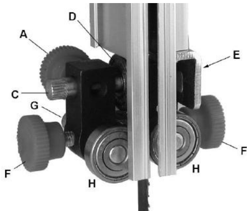
Abb. 25: Obere Sägeblattführungen
