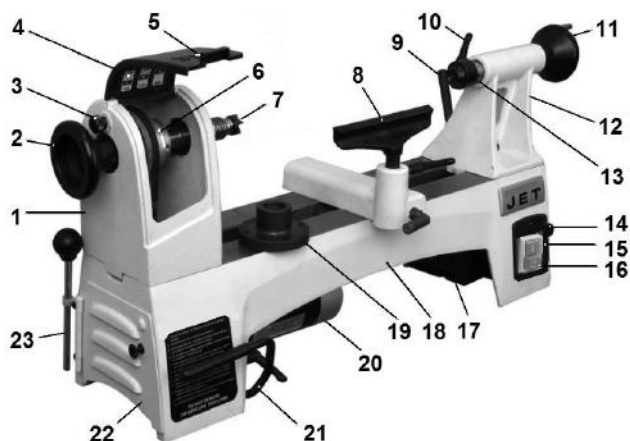
Fig 1 (JWL-1015VS abgebildet)
