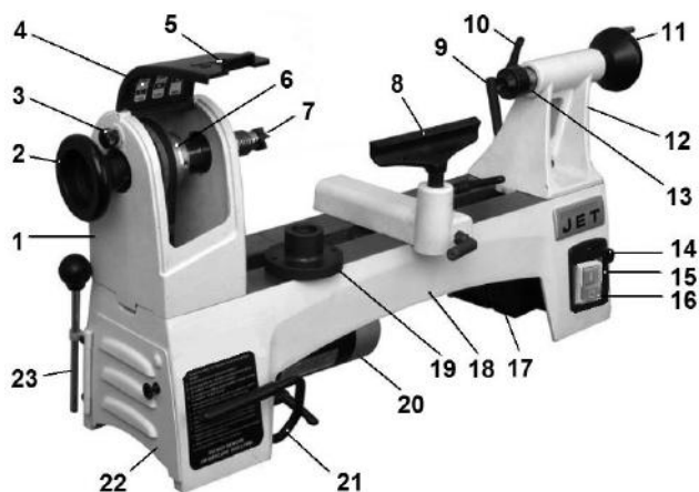
Fig 1 (JWL-1015VS)
