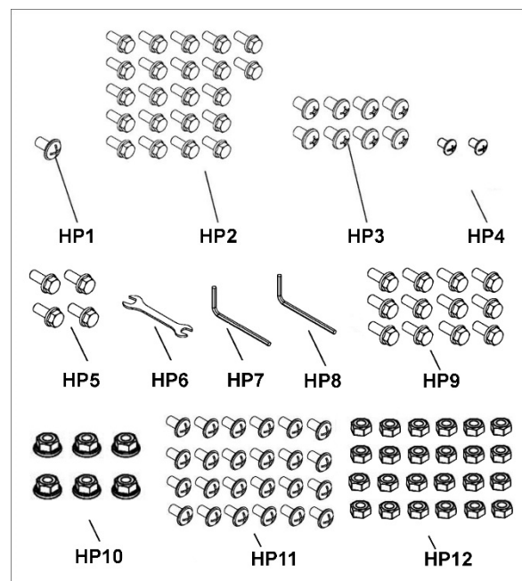
Abb. 2: Inhalt des Hardwarepakets (nicht maßstabsgetreu)
