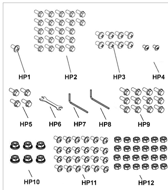
Figure 2 : Contenus de l'emballage du matériel (pas à l'échelle)
